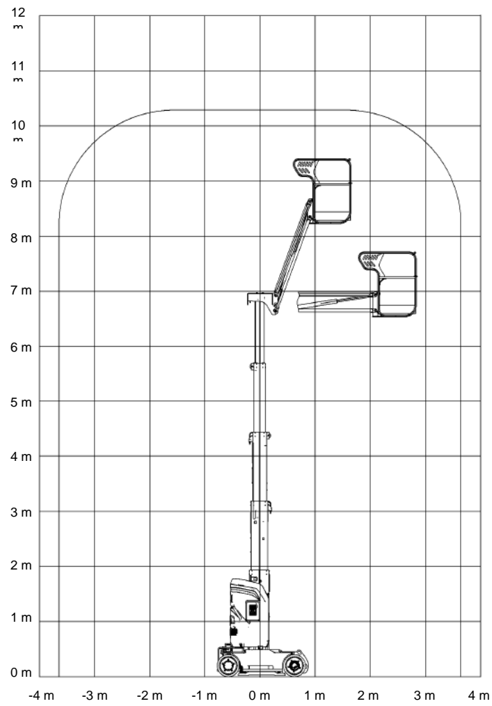
Abbildung 1-1 Arbeitsdiagramm
